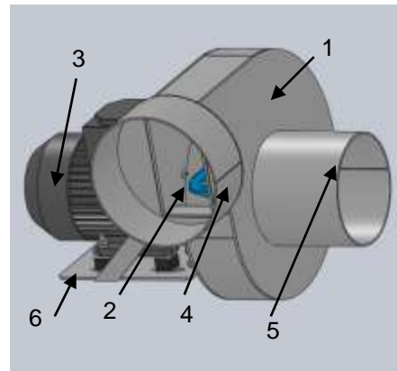
Рисунок 1 - Конструкция дымососа
