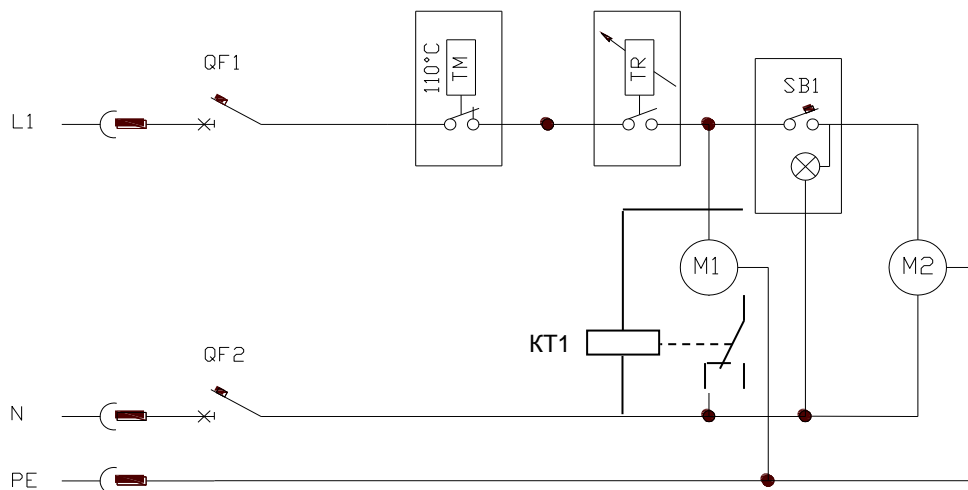
Рисунок 2 - Схема электрическая принципиальная без ПЧВ
